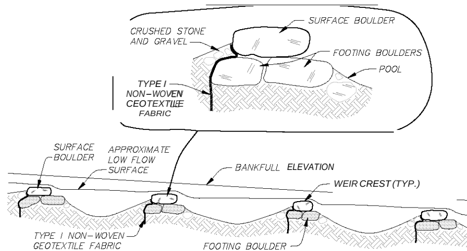
SILT TRAP PROFILE- A-A'
